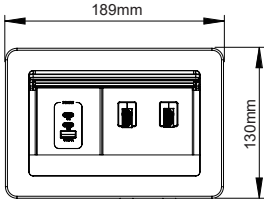
型号:CLB-B062-6000 配置:1个65W氮化镓适配器 2个抽线结构
