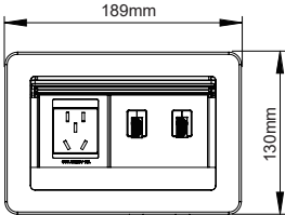
型号:CLB-B062-1100 配置:1个滑动电源 2个抽线结构
